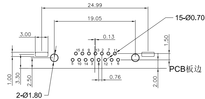
P.C.B LAYOUT
