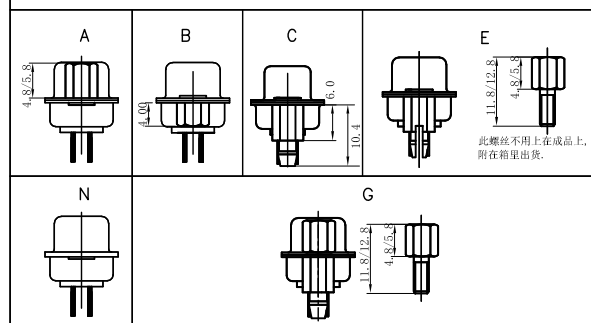
铆钉型式说明
