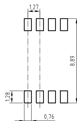
焊盘尺寸：
